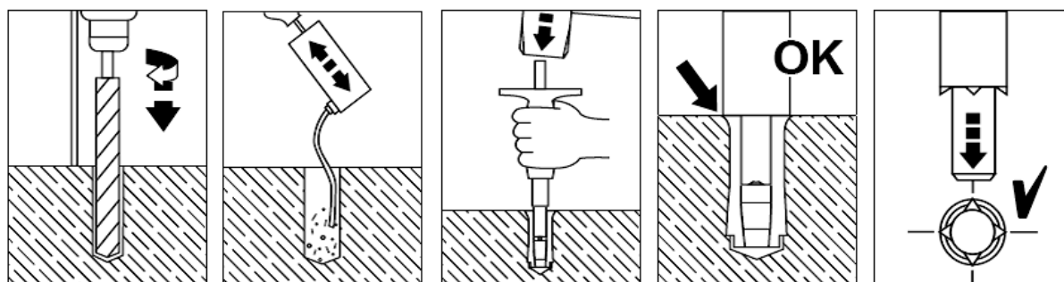
アンカーをセッティングするための手引き。出典：Hilti 社
